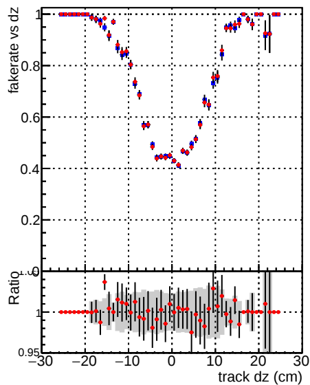
Fake rate vs d DQM CKF XiMinusNOPU_base DQM CKF XiMinusNOPU_retrainOldFiles125_v2_prelimWPM_epoch0
