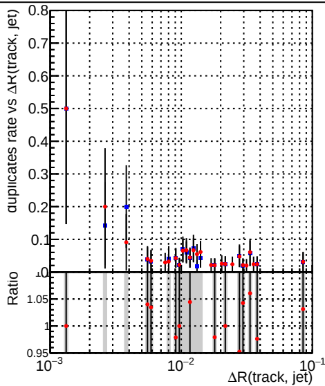
—•— DQM_CKF_XiMinusNOPU_base —•— DQM_CKF_XiMinusNOPU_retrainOldFiles125_v2_prelimWPM_epoch0
