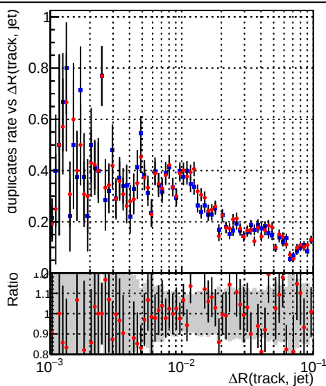
■ DQM_CKF_XiMinusNOPU_base ● DQM_CKF_XiMinusNOPU_retrainOldFiles125_v2_prelimWPM_epoch0
