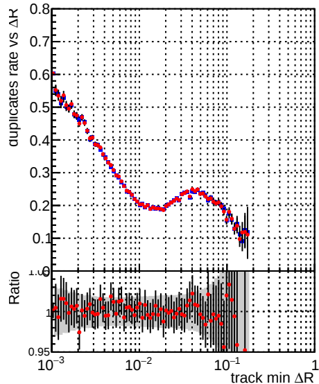
—•— DQM_CKF_XiMinusNOPU_base —•— DQM_CKF_XiMinusNOPU_retrainOldFiles125_v2_prelimWPM_epoch0
