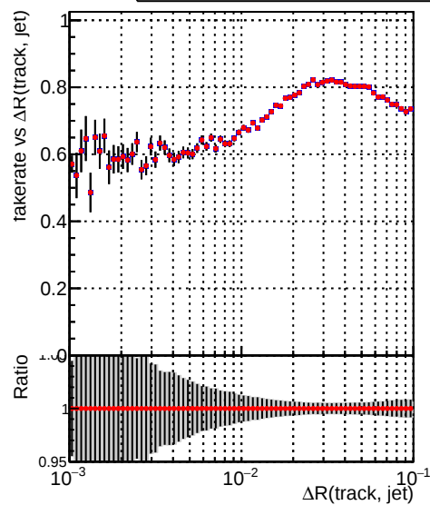
—•— DQM_CKF_XiMinusNOPU_base —•— DQM_CKF_XiMinusNOPU_retrainOldFiles125_v2_prelimWPM_epoch0
