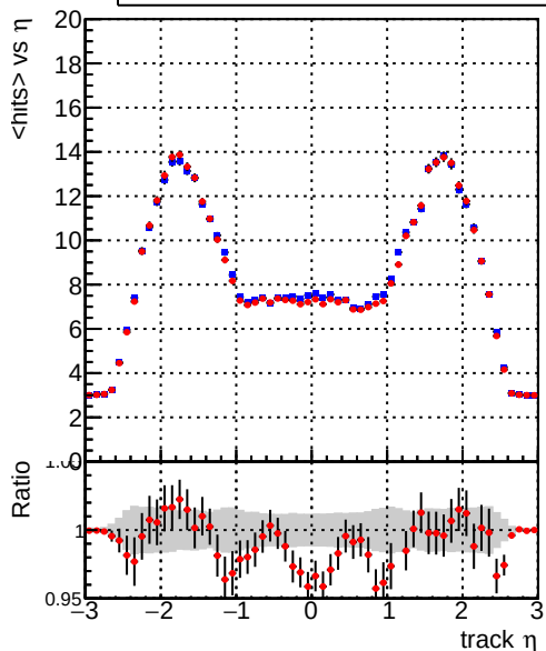
mean hits — DQM_CKF_XiMinusNOPU_base — DQM_CKF_XiMinusNOPU_retrainOldFiles125_v2_prelimWPM_epoch0
