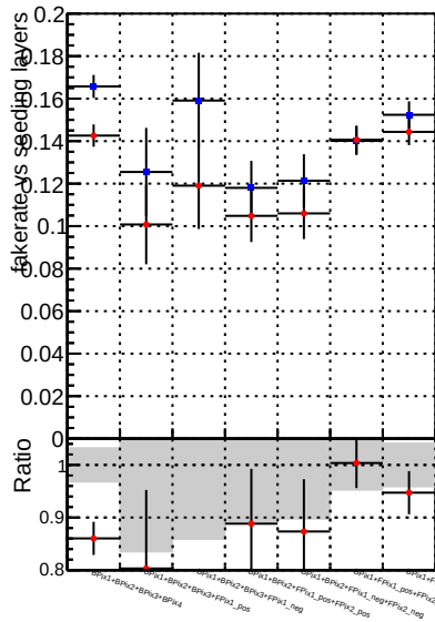
Fake rate vs. ◆ DQM CKF XMinusNOPU_base ● DQM CKF XMinusNOPU_retrainOldFiles125_v2_prelimWPM_epoch0
