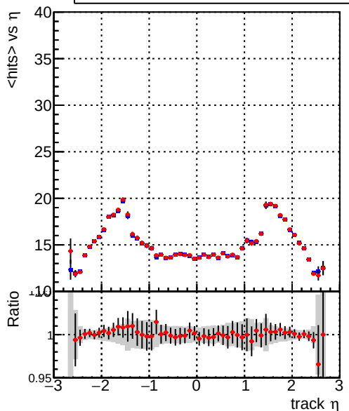
DQM_CKF_XiMinusNOPU_retrainOldFiles125_v2_prelimWPM_epoch0
