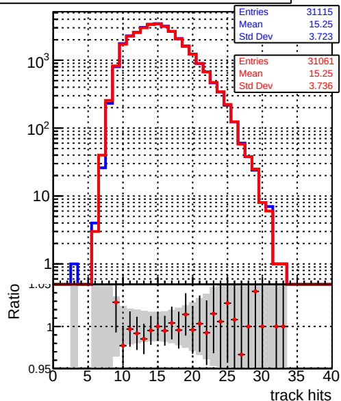
DQM_CKF_XiMinusNOPU_retrainOldFiles125_v2_prelimWPM_epoch0
