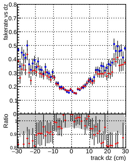
—●— DQM CKF XiMinusNOPU_base —●— DQM CKF XiMinusNOPU_retrainOldFiles125_v2_prelimWPM_epoch0
