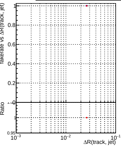
DQM_CKF_XiMinusNOPU_base DQM_CKF_XiMinusNOPU_retrainOldFiles125_v2_prelimWPM_epoch0
