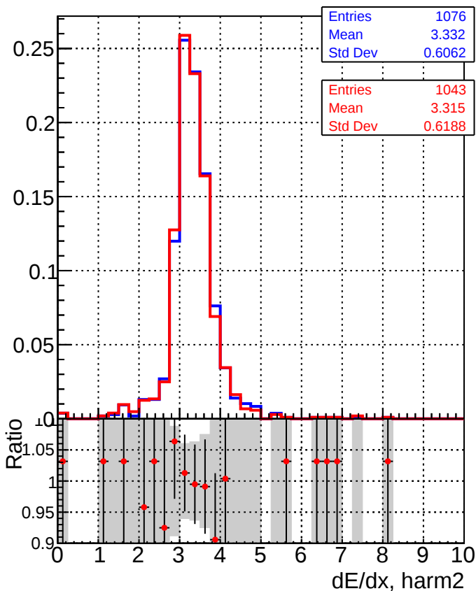
■ DQM_CKF_XiMinusNOPU_base ● DQM_CKF_XiMinusNOPU_retrainOldFiles125_v2_prelimWPM_epoch0
