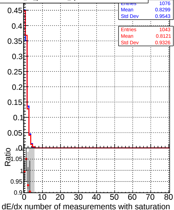
■ DQM_CKF_XiMinusNOPU_base ● DQM_CKF_XiMinusNOPU_retrainOldFiles125_v2_prelimWPM_epoch0
