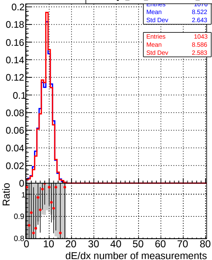
■ DQM_CKF_XiMinusNOPU_base ● DQM_CKF_XiMinusNOPU_retrainOldFiles125_v2_prelimWPM_epoch0
