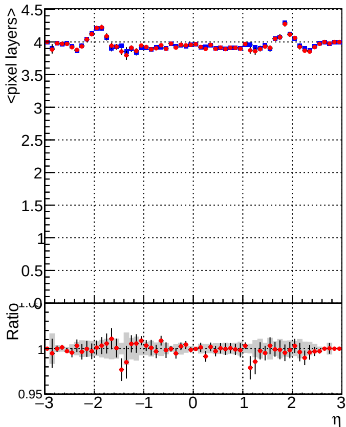
■ DQM_CKF_XiMinusNOPU_base ● DQM_CKF_XiMinusNOPU_retrainOldFiles125_v2_prelimWPM_epoch0
