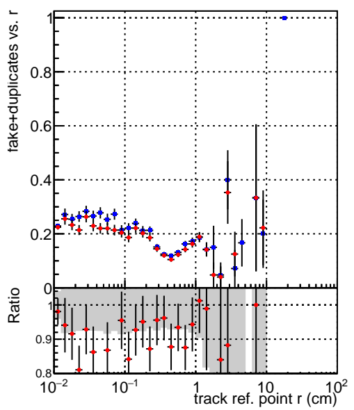
■ DQM_CKF_XiMinusNOPU_base ★ DQM_CKF_XiMinusNOPU_retrainOldFiles125_v2_prelimWPM_epoch0
