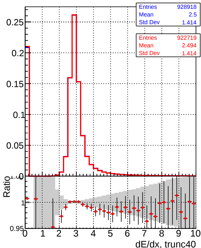
—■— DQM_CKF_XiMinusNOPU_base —●— DQM_CKF_XiMinusNOPU_retrainOldFiles125_v2_prelimWPM_epoch0
