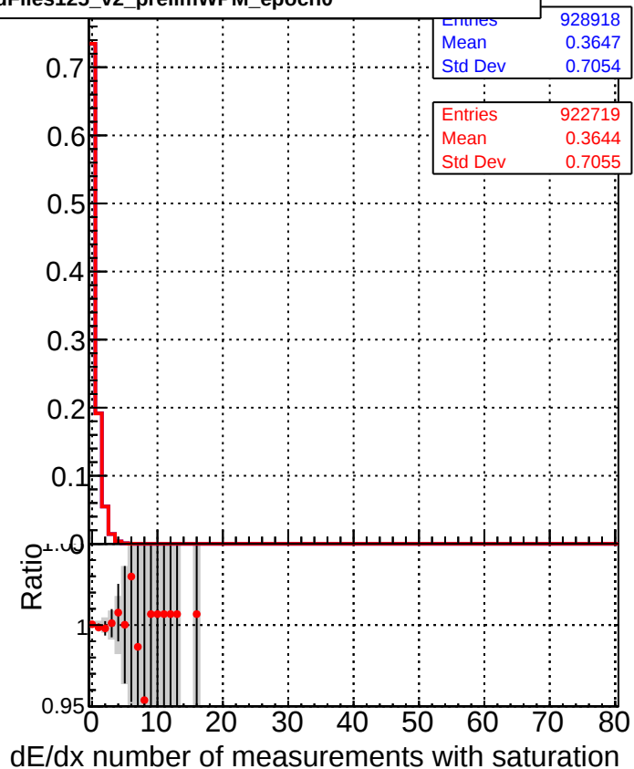
—■— DQM_CKF_XiMinusNOPU_base —●— DQM_CKF_XiMinusNOPU_retrainOldFiles125_v2_prelimWPM_epoch0
