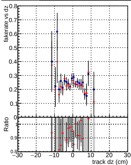
—●— DQM_CKF_XiMinusNOPU_base —●— DQM_CKF_XiMinusNOPU_retrainOldFiles125_v2_prelimWPM_epoch0
