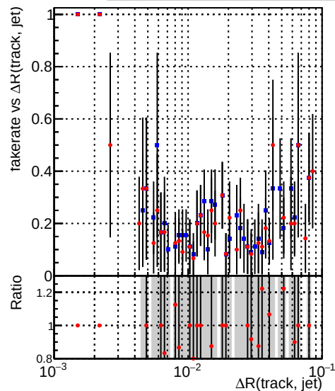
—•— DQM_CKF_XiMinusNOPU_base —•— DQM_CKF_XiMinusNOPU_retrainOldFiles125_v2_prelimWPM_epoch0
