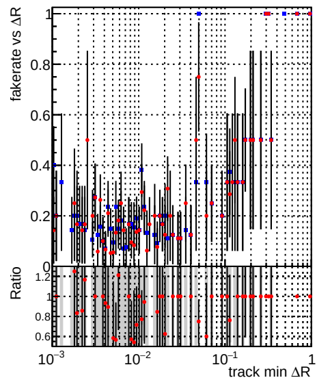
—•— DQM_CKF_XiMinusNOPU_base —•— DQM_CKF_XiMinusNOPU_retrainOldFiles125_v2_prelimWPM_epoch0
