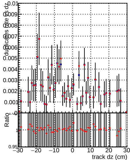
—●— DQM_CKF_XiMinusNOPU_base —●— DQM_CKF_XiMinusNOPU_retrainOldFiles125_v2_prelimWPM_epoch0
