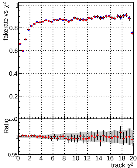
Fake rate vs. \chi^2 —•— DQM CKF XiMinusNOPU_base —•— DQM CKF XiMinusNOPU_retrainOldFiles125_v2_prelimWPM_epoch0
