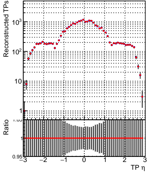
— DQM_CKF_XiMinusNOPU_base — DQM_CKF_XiMinusNOPU_retrainOldFiles125_v2_prelimWPM_epoch0
