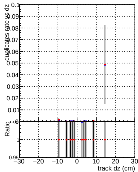
—●— DQM_CKF_XiMinusNOPU_base —●— DQM_CKF_XiMinusNOPU_retrainOldFiles125_v2_prelimWPM_epoch0
