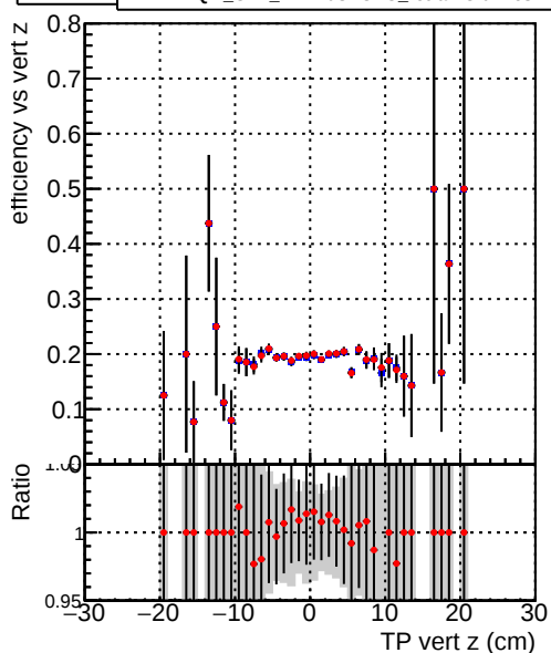
Efficiency vs. TP vert z —●— DQM_CKF_XiMinusNOPU_base —●— DQM_CKF_XiMinusNOPU_retrainOldFiles125_v2_prelimWPM_epoch0
