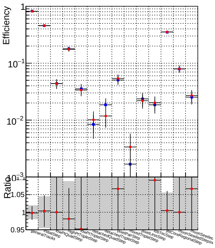
DQM_CKF_XiMinusNOPU_base DQM_CKF_XiMinusNOPU_retrainOldFiles125_v2_prelimWPM_epoch0
