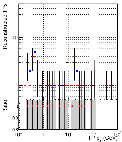
—●— DQM_CKF_XiMinusNOPU_base —●— DQM_CKF_XiMinusNOPU_retrainOldFiles125_v2_prelimWPM_epoch0
