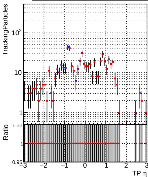
—●— DQM_CKF_XiMinusNOPU_base —●— DQM_CKF_XiMinusNOPU_retrainOldFiles125_v2_prelimWPM_epoch0
