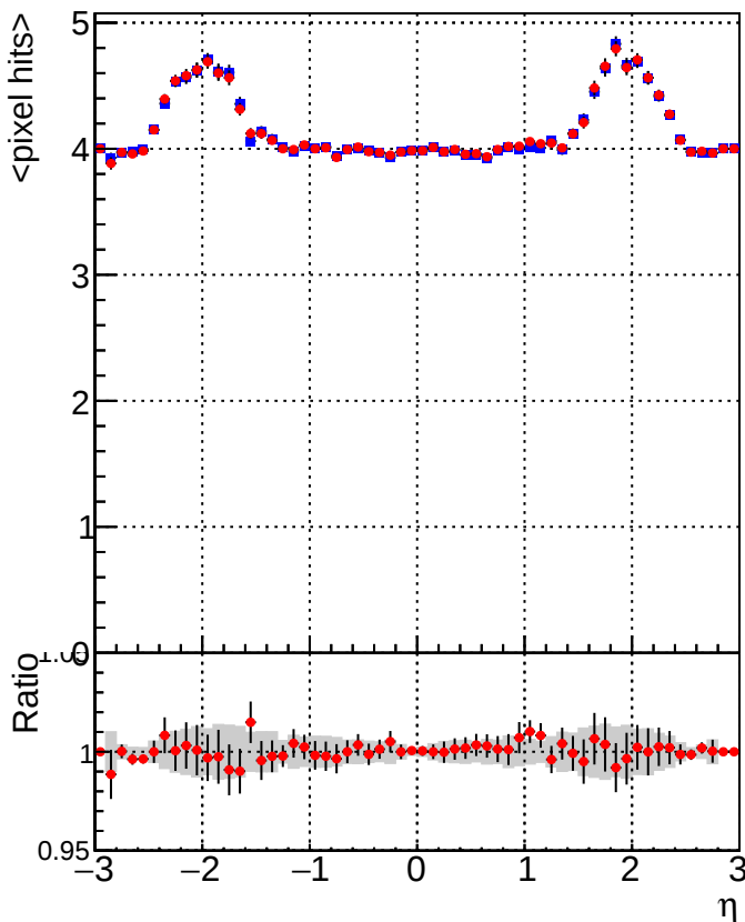
■ DQM_CKF_XiMinusNOPU_base ● DQM_CKF_XiMinusNOPU_retrainOldFiles125_v2_prelimWPM_epoch0
