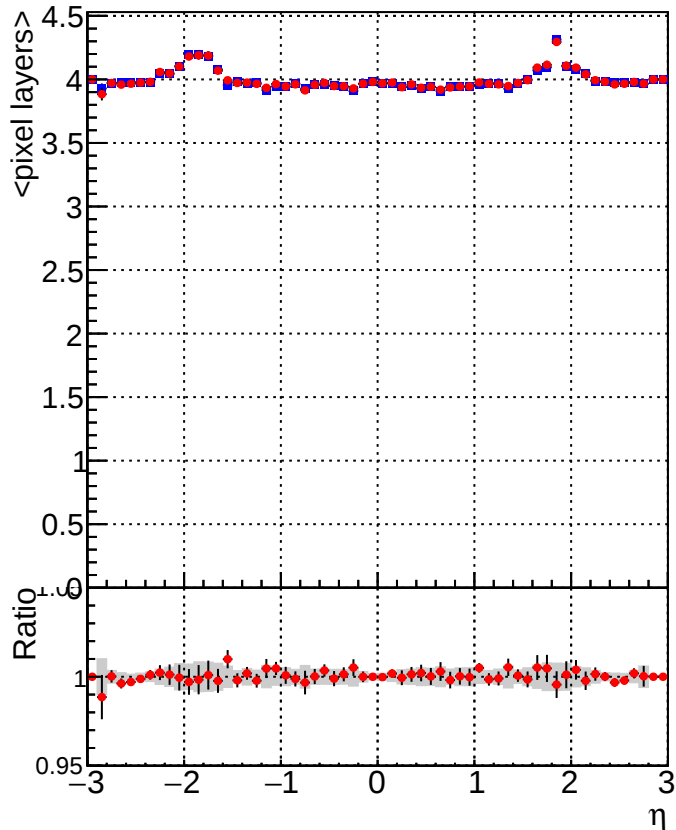
■ DQM_CKF_XiMinusNOPU_base ● DQM_CKF_XiMinusNOPU_retrainOldFiles125_v2_prelimWPM_epoch0
