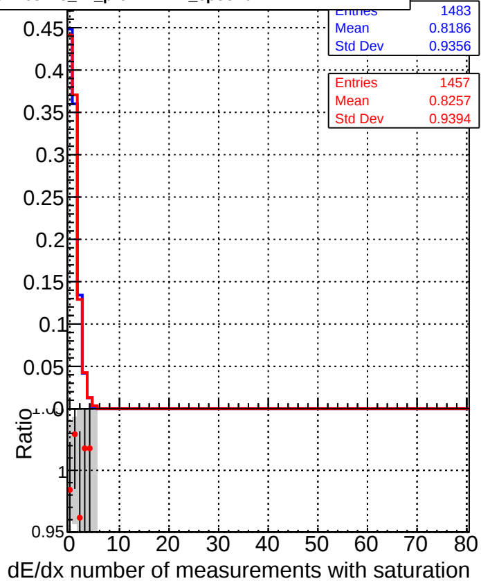
DQM_CKF_XiMinusNOPU_base DQM_CKF_XiMinusNOPU_retrainOldFiles125_v2_prelimWPM_epoch0
