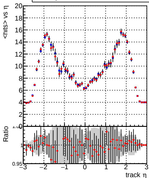
mean hits — DQM_CKF_XiMinusNOPU_base — DQM_CKF_XiMinusNOPU_retrainOldFiles125_v2_prelimWPM_epoch0
