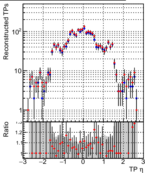
DQM_CKF_XiMinusNOPU_base DQM_CKF_XiMinusNOPU_retrainOldFiles125_v2_prelimWPM_epoch0
