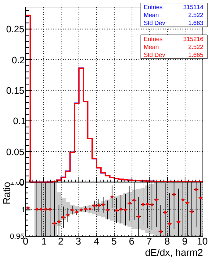
DQM_CKF_XiMinusNOPU_base
