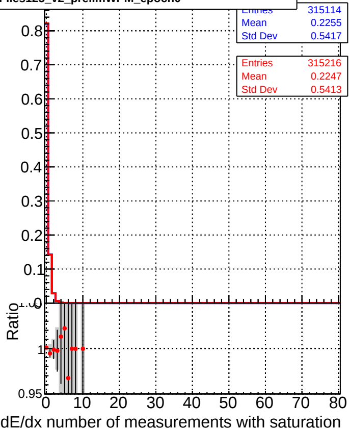
DQM_CKF_XiMinusNOPU_retrainOldFiles125_v2_prelimWPM_epoch0
