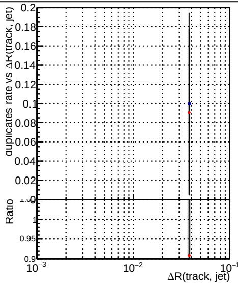
—●— DQM_CKF_XiMinusNOPU_base —●— DQM_CKF_XiMinusNOPU_retrainOldFiles125_v2_prelimWPM_epoch0
