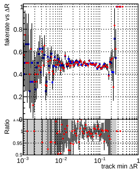
—●— DQM_CKF_XiMinusNOPU_base —●— DQM_CKF_XiMinusNOPU_retrainOldFiles125_v2_prelimWPM_epoch0
