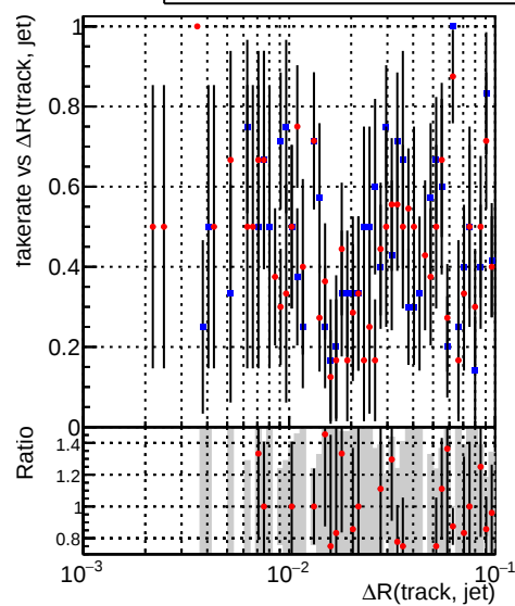
—●— DQM_CKF_XiMinusNOPU_base —●— DQM_CKF_XiMinusNOPU_retrainOldFiles125_v2_prelimWPM_epoch0
