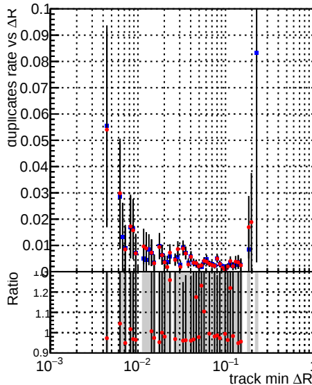
—●— DQM_CKF_XiMinusNOPU_base —●— DQM_CKF_XiMinusNOPU_retrainOldFiles125_v2_prelimWPM_epoch0
