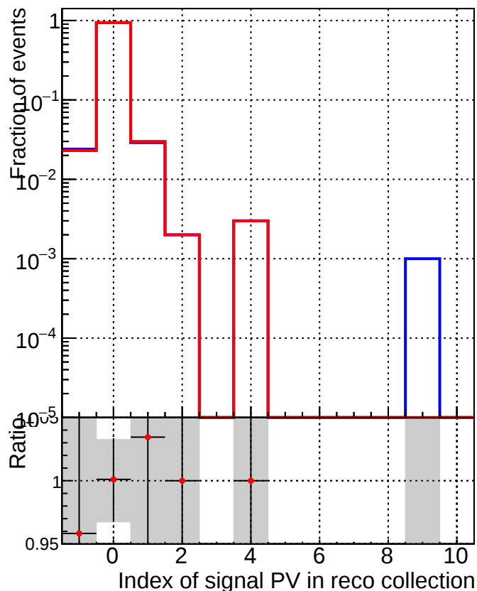
■ DQM_CKF_TTbase ● DQM_CKF_TT_retrainOldFiles125_v2_prelimWPM_epoch4
