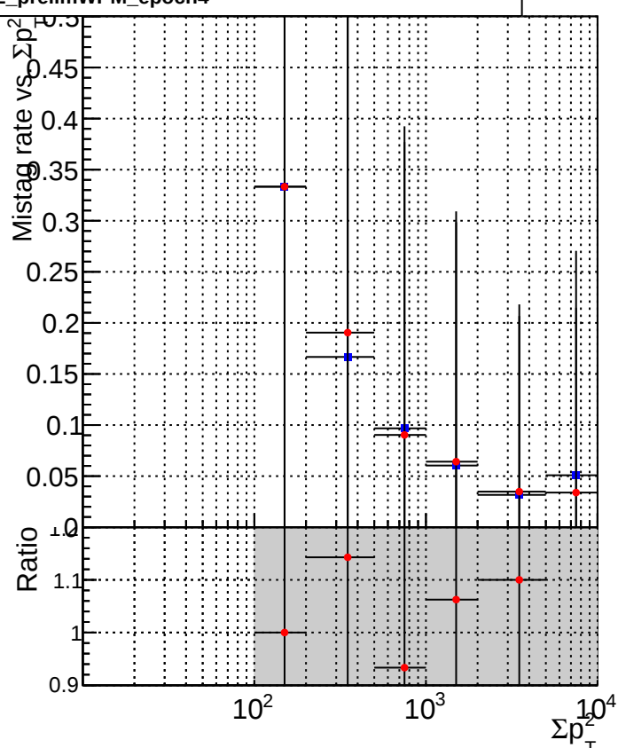
■ DQM_CKF_TTbase ● DQM_CKF_TT_retrainOldFiles125_v2_prelimWPM_epoch4
