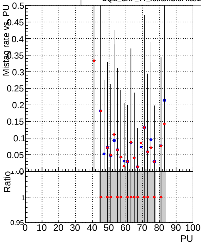
■ DQM_CKF_TTbase ● DQM_CKF_TT_retrainOldFiles125_v2_prelimWPM_epoch4
