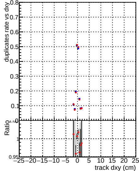
—●— DQM CKF TTbase —●— DQM CKF TT_retrainOldFiles125_v2_prelimWPM_epoch4
