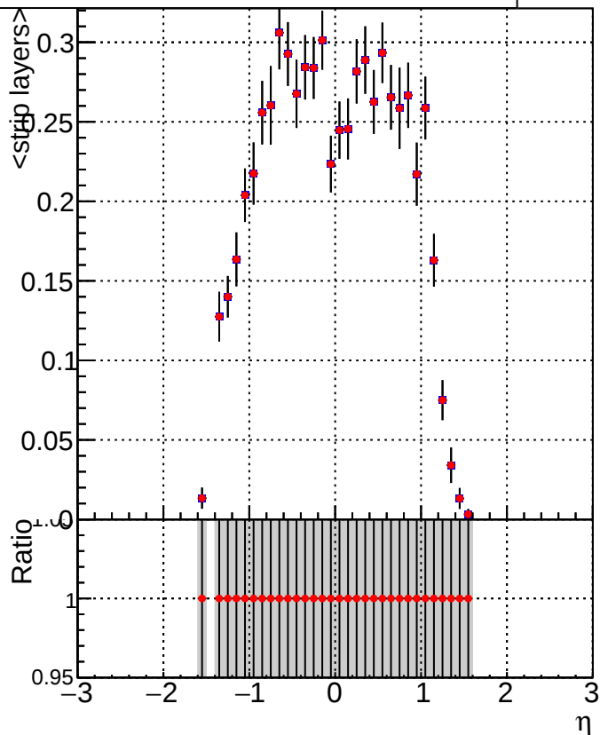
DQM_CKF_TTbase DQM_CKF_TT_retrainOldFiles125_v2_prelimWPM_epoch4
