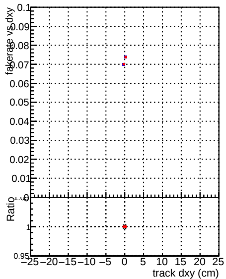
— DQM_CKF_TTbase — DQM_CKF_TT_retrainOldFiles125_v2_prelimWPM_epoch4
