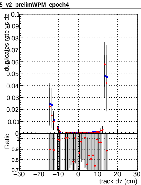
—●— DQM CKF TTbase —●— DQM CKF TT_retrainOldFiles125_v2_prelimWPM_epoch4
