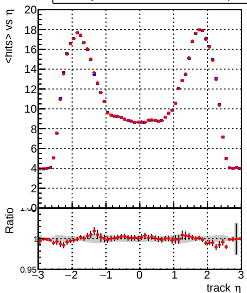
— DQM_CKF_TTbase — DQM_CKF_TT_retrainOldFiles125_v2_prelimWPM_epoch4
