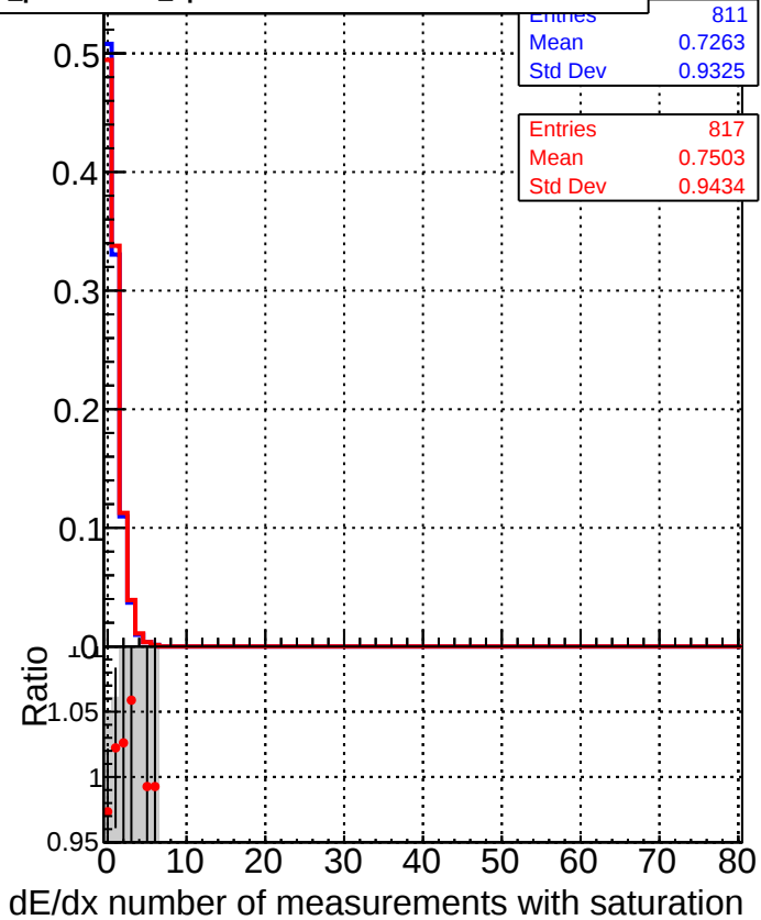
DQM_CKF_TTbase DQM_CKF_TT_retrainOldFiles125_v2_prelimWPM_epoch4
