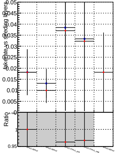
Fake rate vs. - DQM CKF TTbase - DQM CKF TT_retrainOldFiles125_v2_prelimWPM_epoch4
