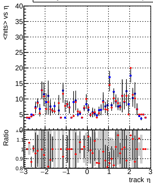
— DQM_CKF_TTbase — DQM_CKF_TT_retrainOldFiles125_v2_prelimWPM_epoch4
