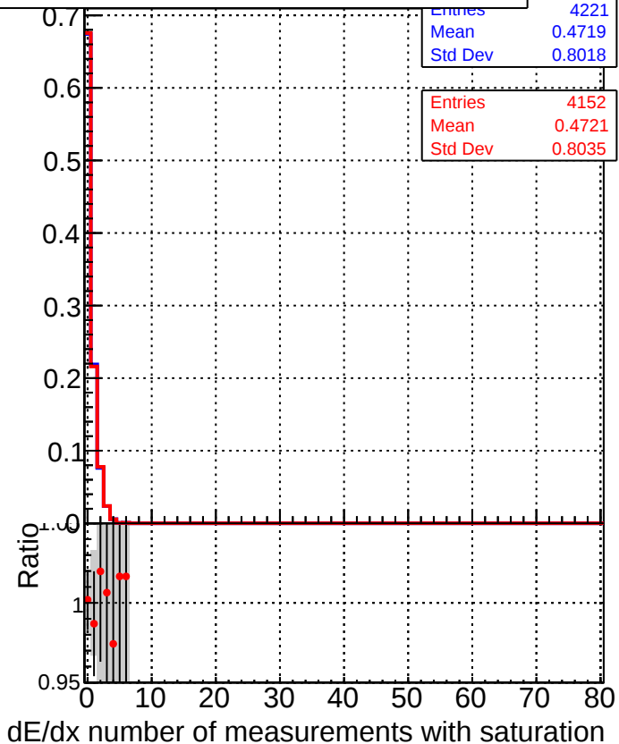
DQM_CKF_TTbase DQM_CKF_TT_retrainOldFiles125_v2_prelimWPM_epoch4
