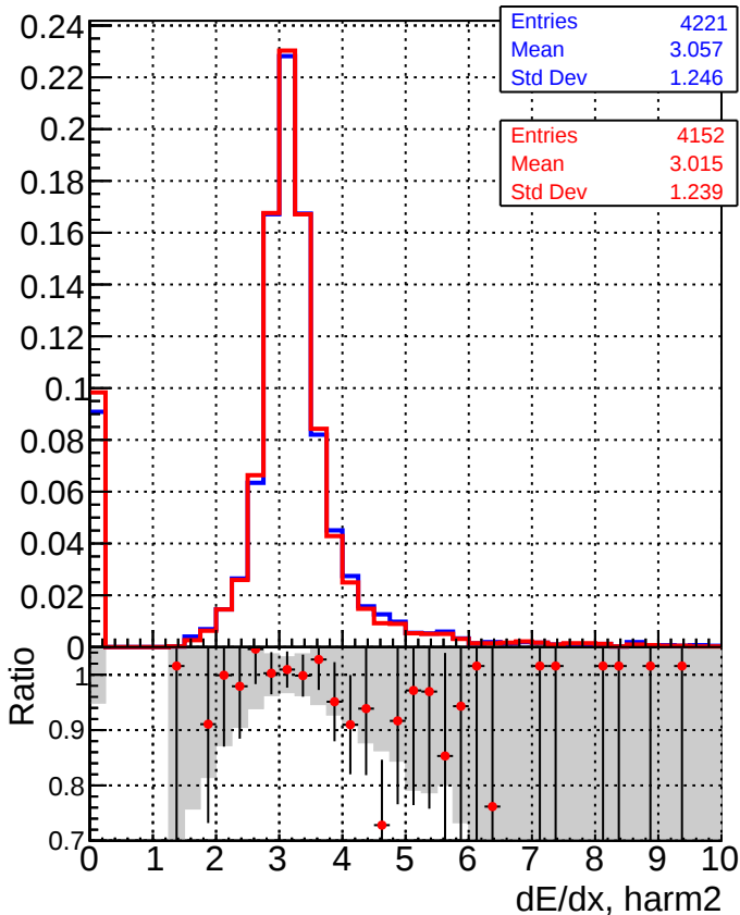
DQM_CKF_TTbase DQM_CKF_TT_retrainOldFiles125_v2_prelimWPM_epoch4
