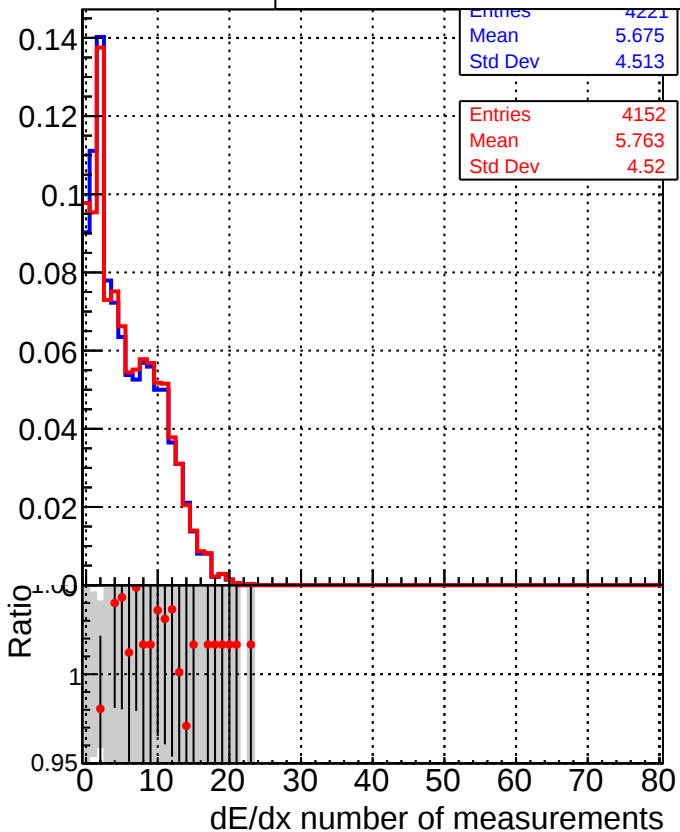
DQM_CKF_TTbase DQM_CKF_TT_retrainOldFiles125_v2_prelimWPM_epoch4
