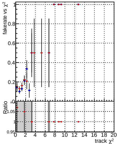
Fake rate vs. —•— DQM CKF TTbase —•— DQM CKF TT_retrainOldFiles125_v2_prelimWPM_epoch4
