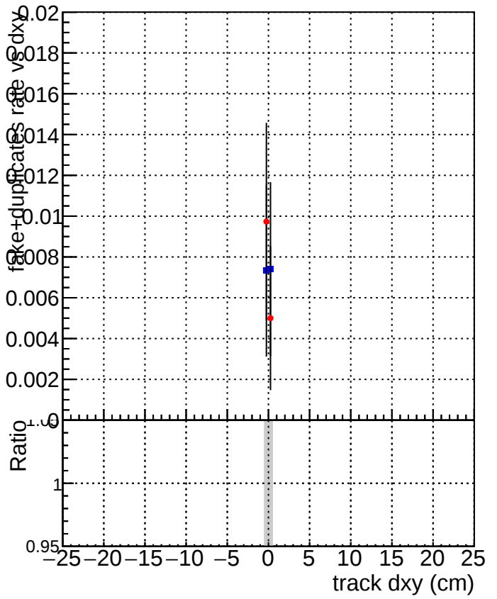
DQM_CKF_TTbase DQM_CKF_TT_retrainOldFiles125_v2_prelimWPM_epoch4
