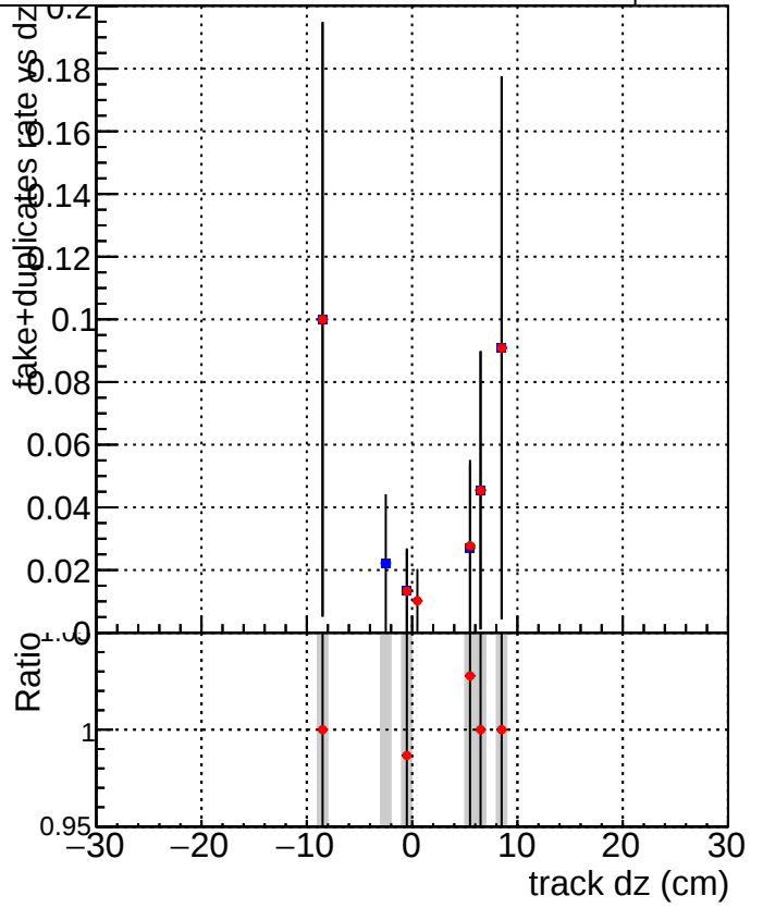
DQM_CKF_TTbase DQM_CKF_TT_retrainOldFiles125_v2_prelimWPM_epoch4
