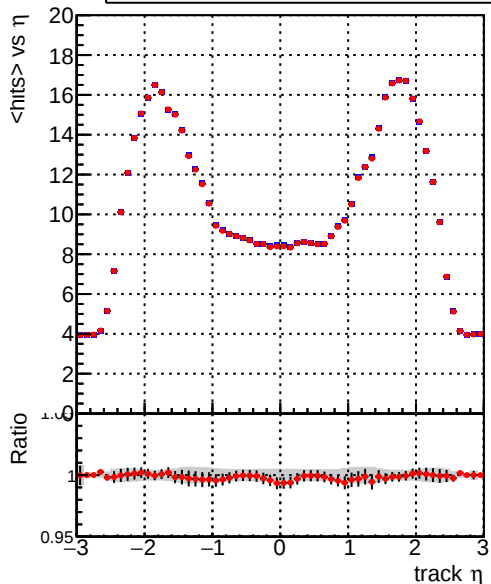
— DQM_CKF_TTbase — DQM_CKF_TT_retrainOldFiles125_v2_prelimWPM_epoch4
