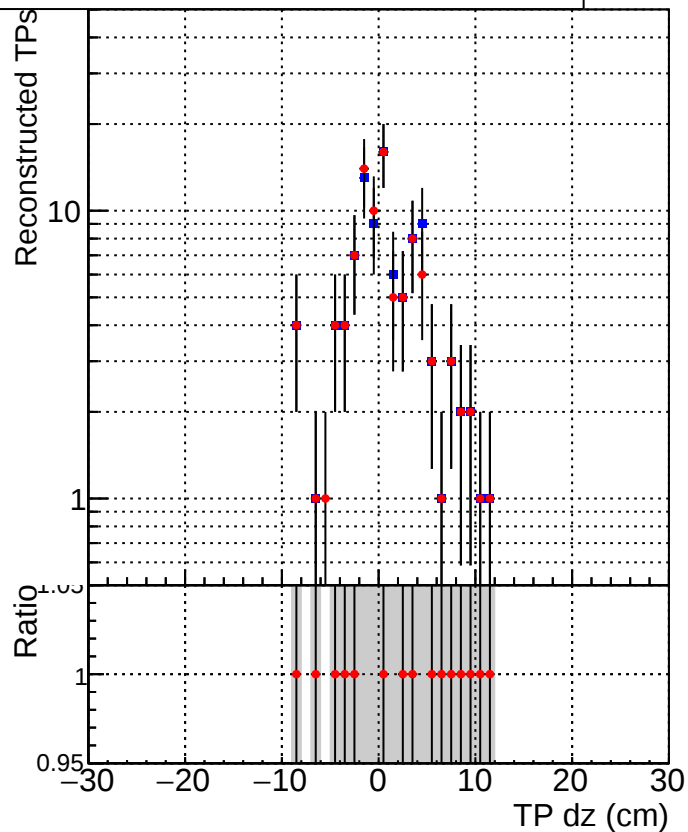
■ DQM_CKF_TTbase ■ DQM_CKF_TT_retrainOldFiles125_v2_prelimWPM_epoch4
