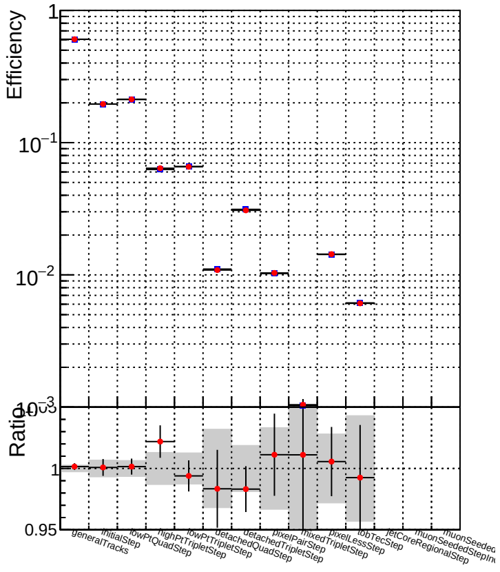
DQM_CKF_TTbase DQM_CKF_TT_retrainOldFiles125_v2_prelimWPM_epoch3
