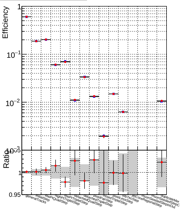
DQM_CKF_TTbase DQM_CKF_TT_retrainOldFiles125_v2_prelimWPM_epoch3
