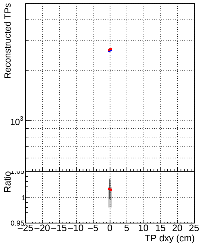
■ DQM_CKF_TTbase ■ DQM_CKF_TT_retrainOldFiles125_v2_prelimWPM_epoch3
