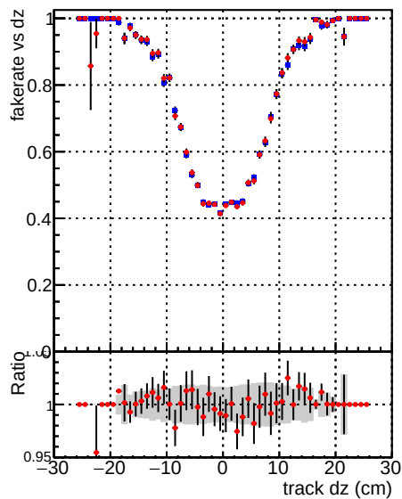
—●— DQM CKF TTbase —●— DQM CKF TT_retrainOldFiles125_v2_prelimWPM_epoch3
