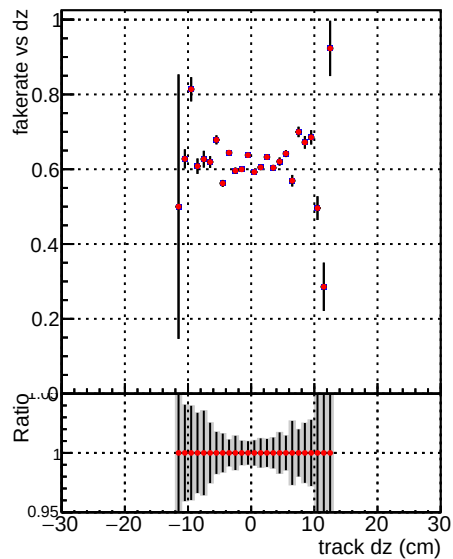
Fake rate vs dz DQM CKF TTbase DQM CKF TT_retrainOldFiles125_v2_prelimWPM_epoch3
