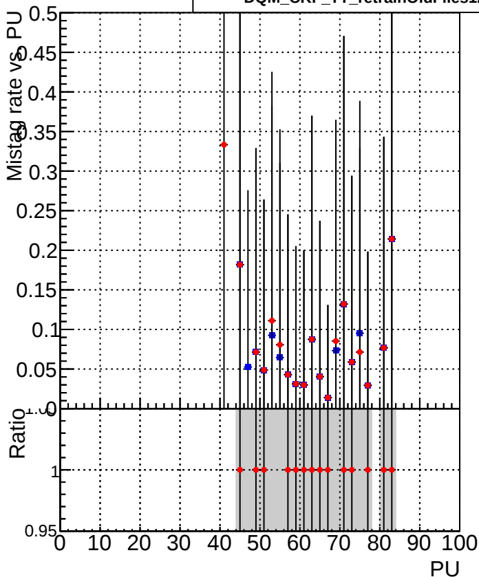
■ DQM_CKF_TTbase ● DQM_CKF_TT_retrainOldFiles125_v2_prelimWPM_epoch3
