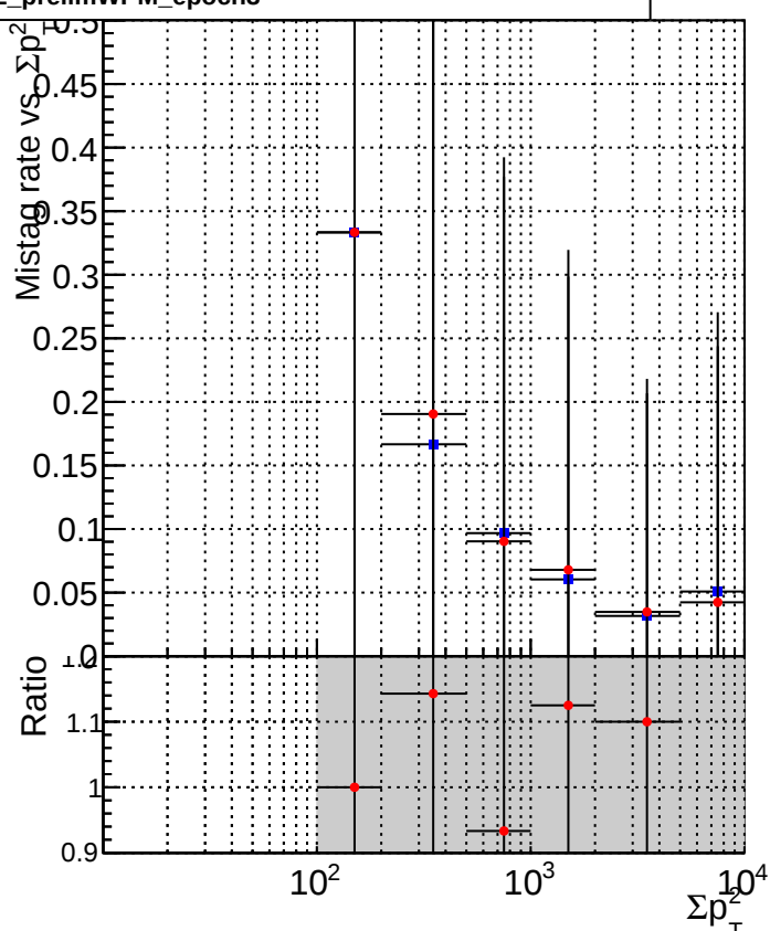
■ DQM_CKF_TTbase ● DQM_CKF_TT_retrainOldFiles125_v2_prelimWPM_epoch3
