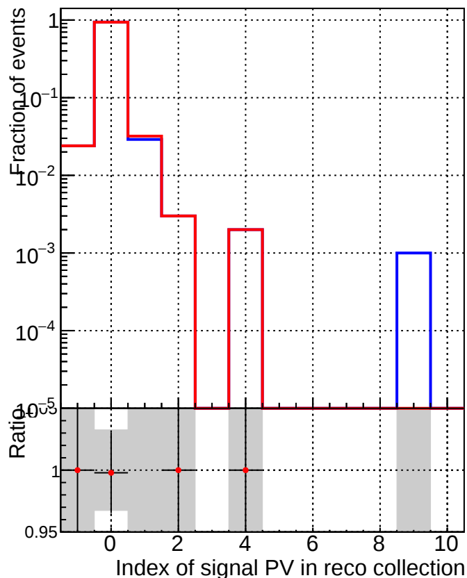
■ DQM_CKF_TTbase ● DQM_CKF_TT_retrainOldFiles125_v2_prelimWPM_epoch3
