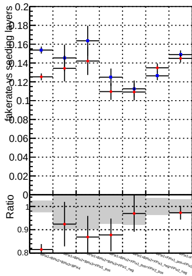
Fake rate vs. —•— DQM CKF TTbase —•— DQM CKF TT_retrainOldFiles125_v2_prelimWPM_epoch3
