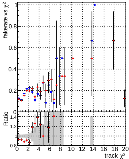
Fake rate vs. —•— DQM CKF TTbase —•— DQM CKF TT_retrainOldFiles125_v2_prelimWPM_epoch3
