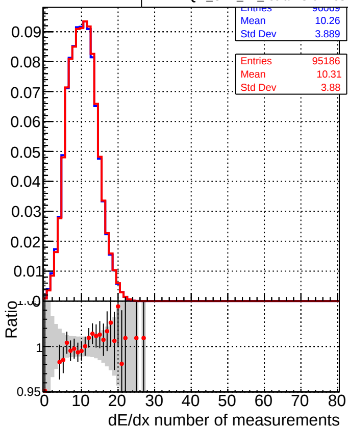
█ DQM_CKF_TTbase —●— DQM_CKF_TT_retrainOldFiles125_v2_prelimWPM_epoch3
